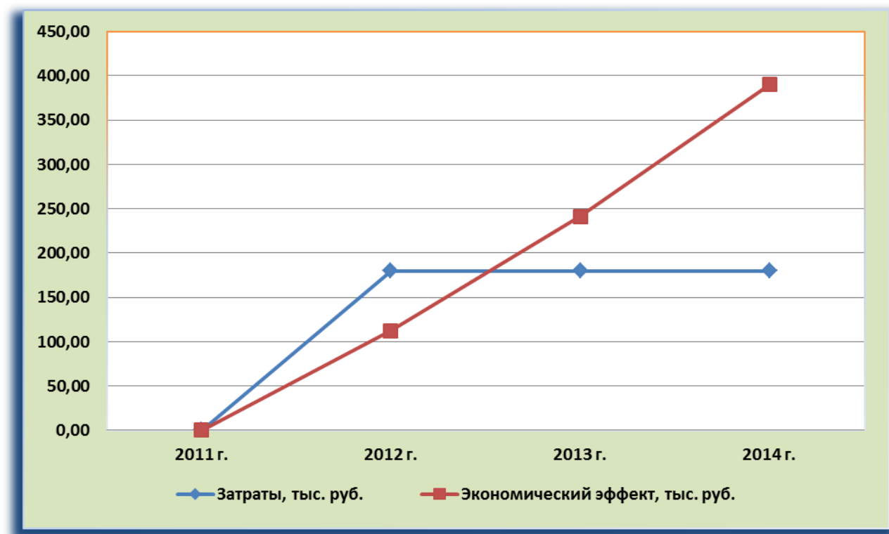
Диаграмма 1 Экономический эффект от замены светильников с лампами ДРЛ на более энергоэффективные светильники с лампами ДНАТ
